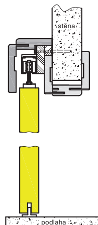
Posuv po stěně s použitím průchozí obložkové zárubně (záklap 80mm)
