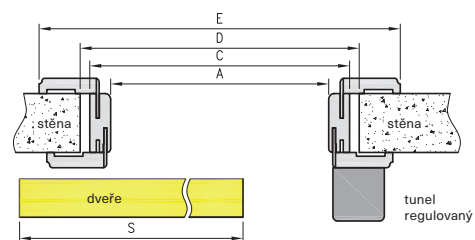
Průřez horizontální (systém levý)
