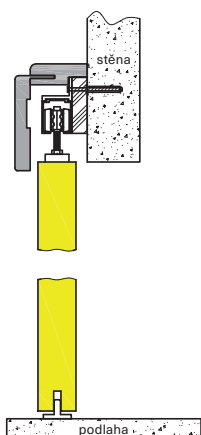
Posuv po stěně bez použití průchozí obložkové zárubně
