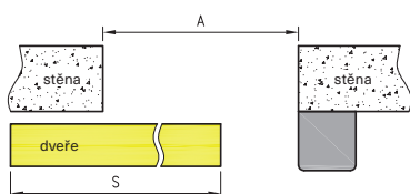
Průřez horizontální (systém levý)
