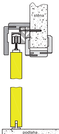
Posuv po stěně s použitím průchozí obložkové zárubně (záklap 63mm)
