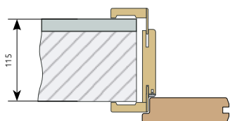
obl. zárubeň B (95-115 mm) síla stěny 115 mm záklopový límeček vysunutý v rozsahu regulace 0-20 mm na své maximum.
