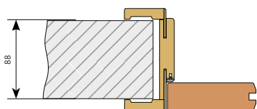
obl. zárubeň B (88-108 mm) síla stěny 90 mm zasunutý záklopový límeč
