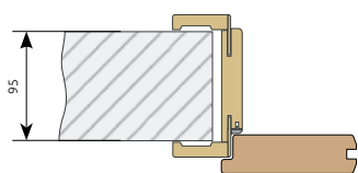
obl. zárubeň B (95-115 mm) síla stěny 95 mm zasunutý záklopový límeček
