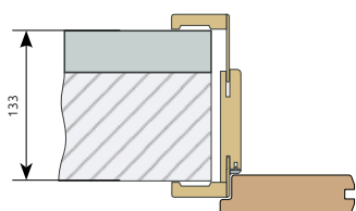
obl. zárubeň B (95-115 mm) síla stěny 133 mm záklopový límeček s delším spojovacím perem +18 mm
