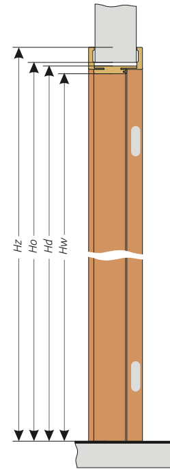
Rozměry obložení bezpodrážkového systému
