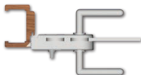
obr. 1 - dveře pravé / knoflík z vnějšku
